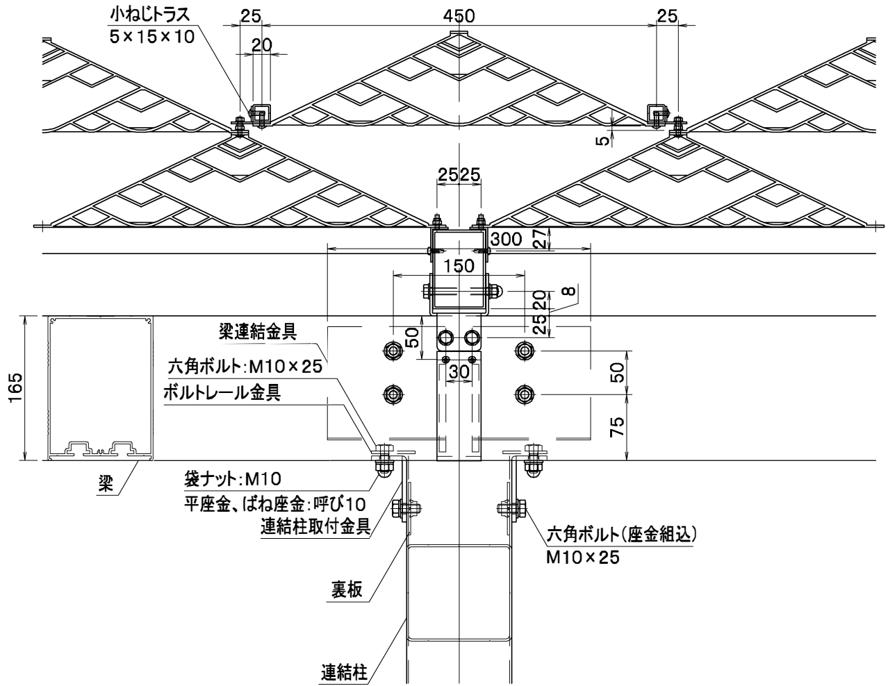
間口連棟部 正面図
