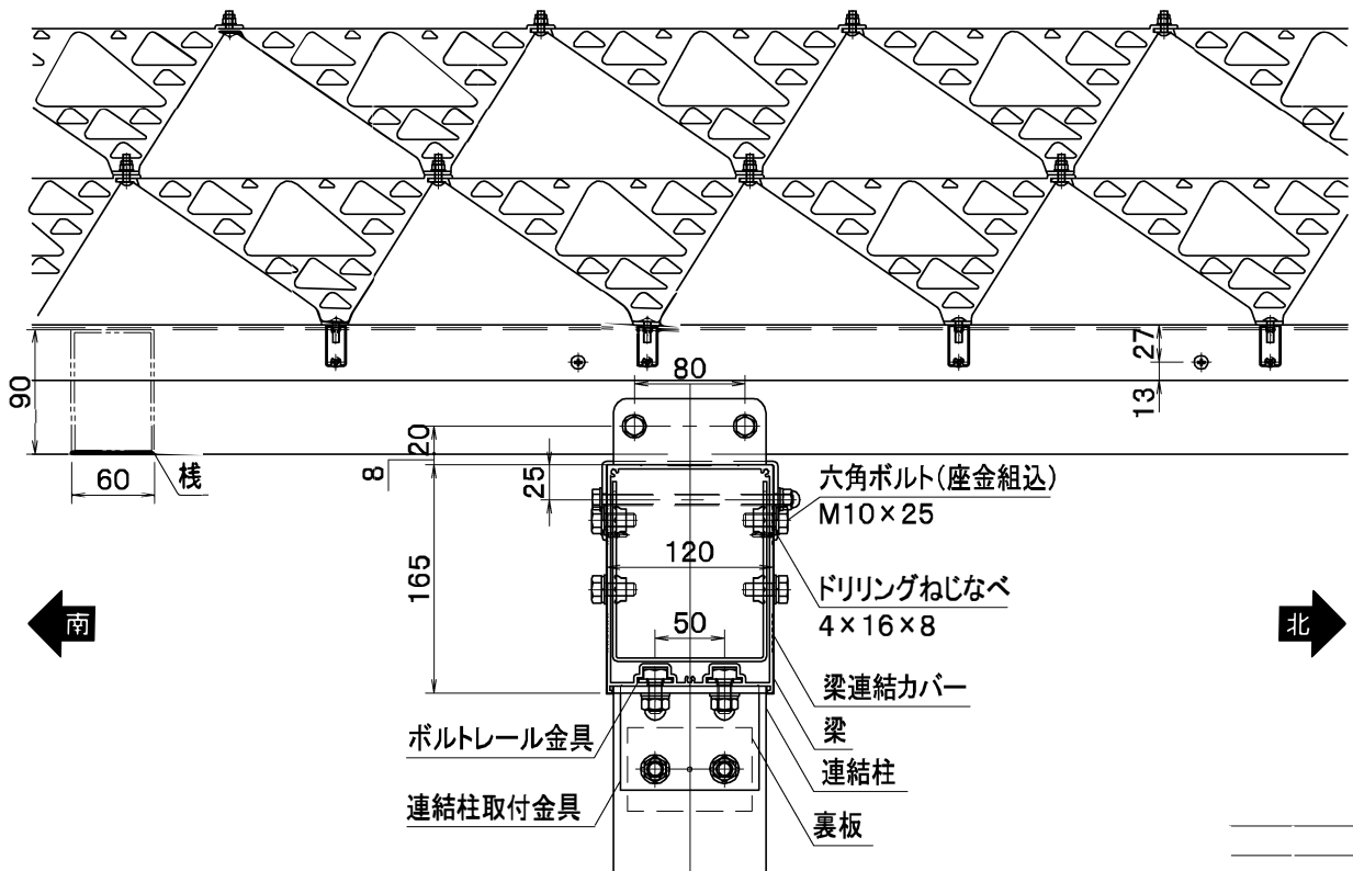
間口連棟部 側面図
